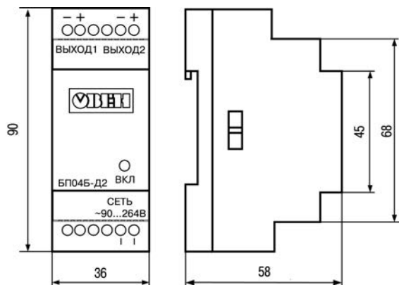
Рисунок 3.1 – Габаритные размеры блока питания БП04Б-Д2-х
