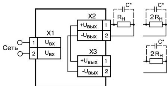
Рисунок 5.1 – Типовая схема подключения блока питания БП04Б - Д2 – Х
