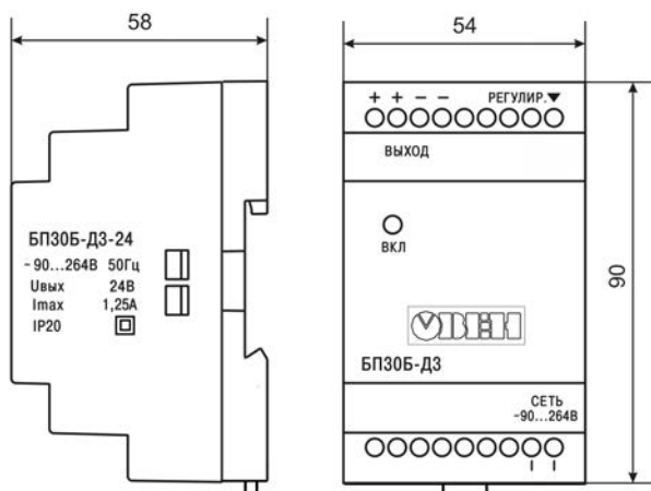
Рисунок 3.1 – Габаритные размеры блока
