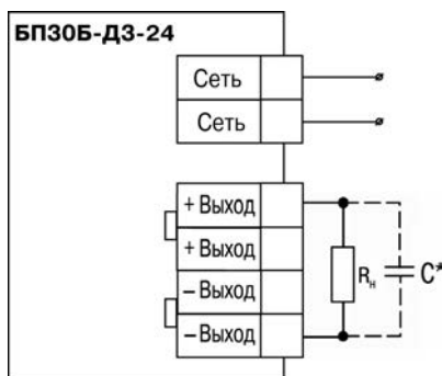
Рисунок 5.1 – Типовая схема подключения блока
