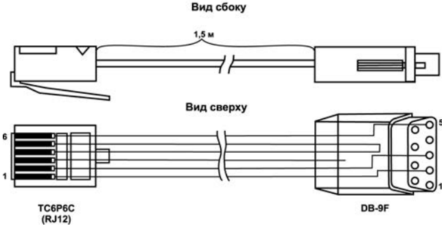
Рисунок Д.1 – Схема кабеля КС1
