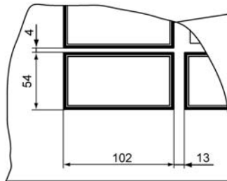
Рисунок А.6 - Прибор в корпусе Щ2, установленный в щит толщиной 3 мм
