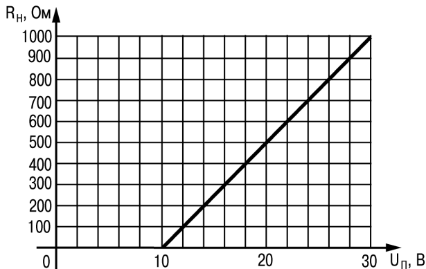
Рисунок 3.16 – График зависимости R_{н} ( U_{п} )
