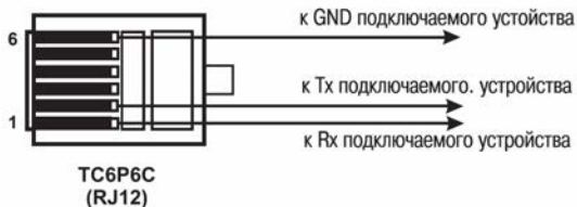
Рисунок Б.4 - Схема кабеля для подключения к порту Debug RS-232
