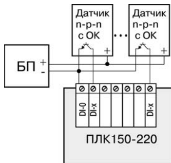
Рисунок Б.5 - Схема подключения к ПЛК150 дискретных датчиков с полупроводниковым выходным каскадом
