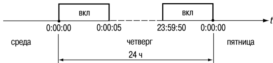
Рисунок Б.2 – Диаграмма включения выхода блока
