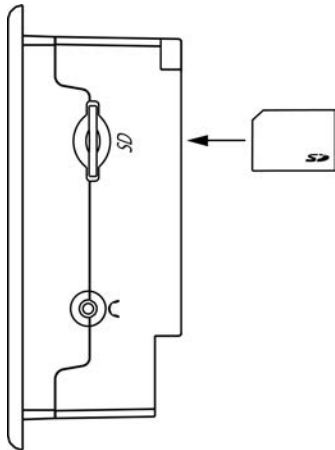
Рисунок 3.3 – Внешний вид боковой панели
