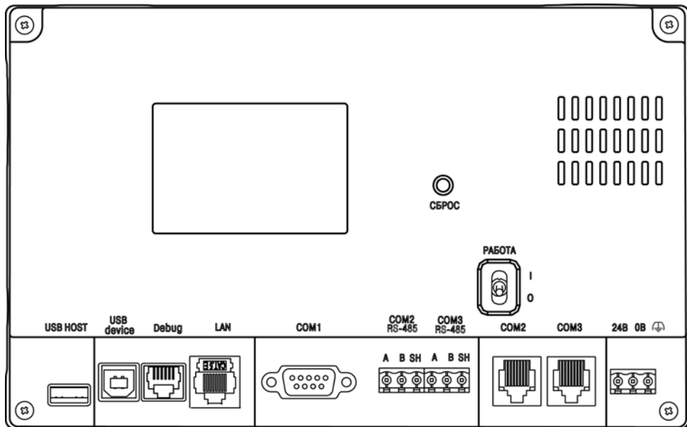
Рисунок 3.2 – Внешний вид задней панели СПК207-XX.03
