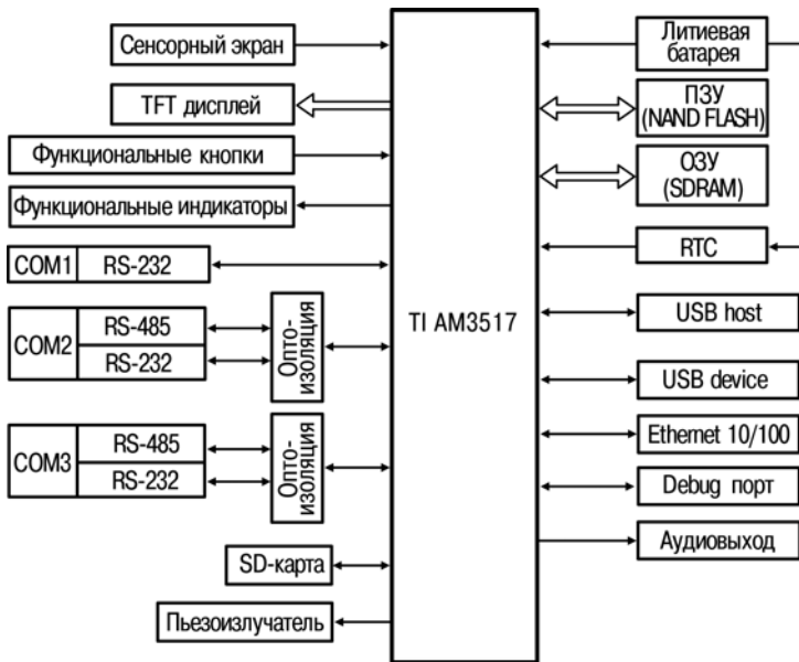
Рисунок 3.5 – Структурная схема панели
