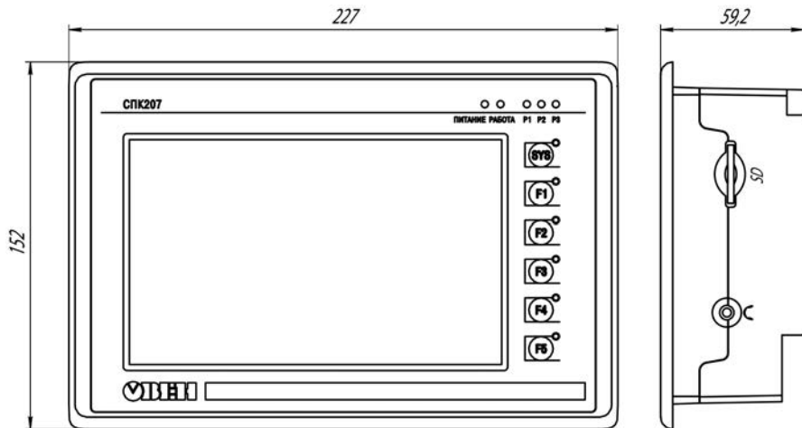
Рисунок А.1 – Габаритные размеры
